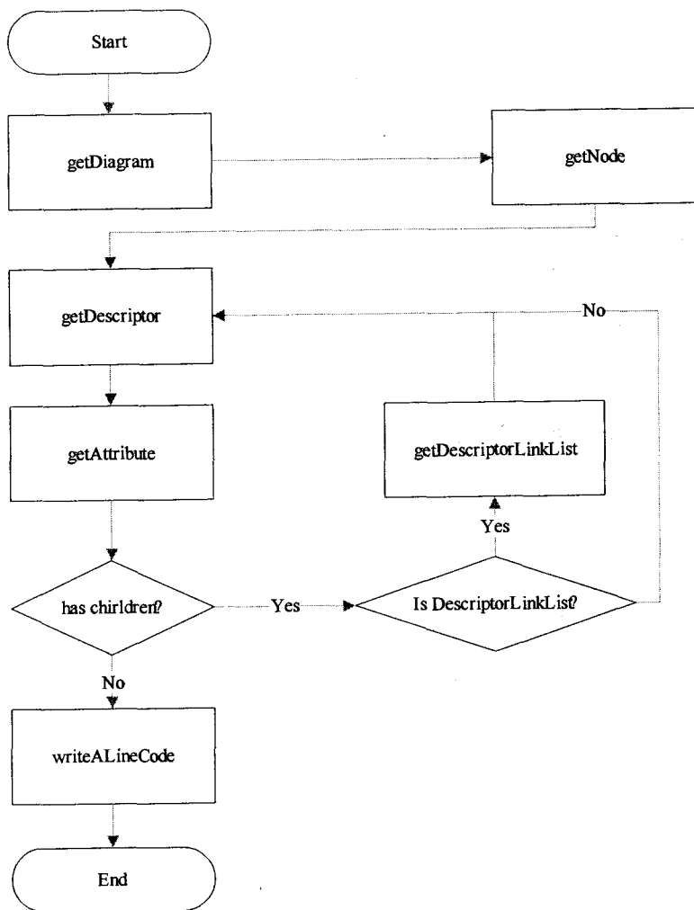
图4 解析文件生成代码的流程
