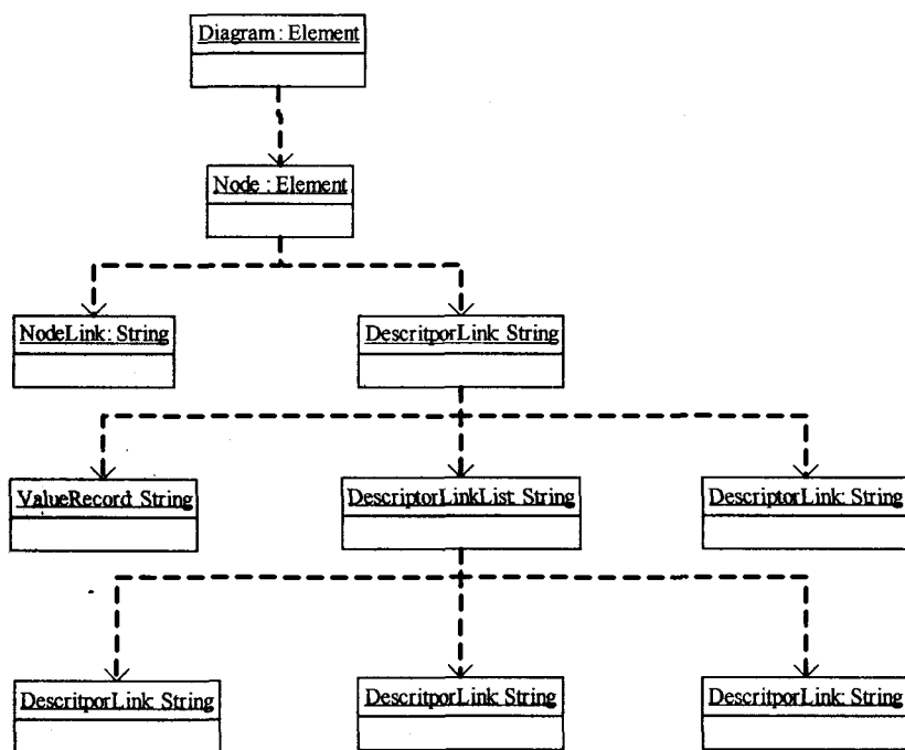
图 2 被测试数据层次结构
