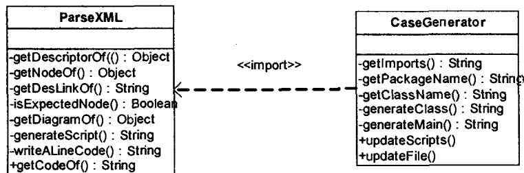
图 3 ParseXML 与 CaseGenerator 类结构与关系
