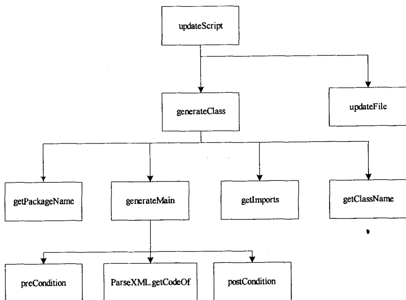
图5 CaseGenerator 类中方法调用关系
