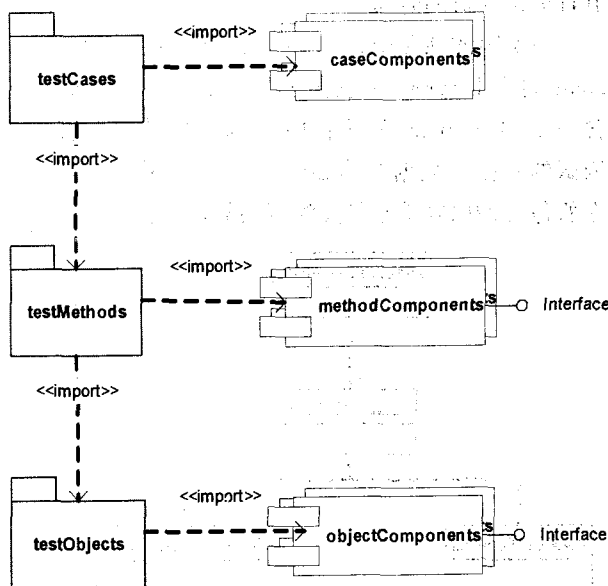
图1 三层测试框架结构示意图
