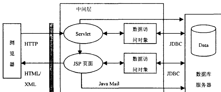
图 1 一种典型的 Web 应用体系结构
